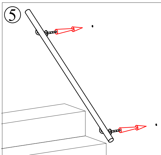
Osazení madla
